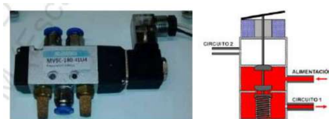
Figura. 5-12 Electroválvula selectora
