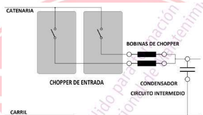
Figura 1-55. Chopper bifásico.
