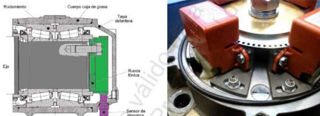
Figura. 2-70 Odómetros. Inductivo (izquierda) y óptico (derecha)
