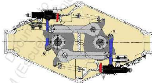
Figura 6-31 Armados
