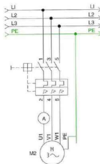
↑ Figura 4.35. Esquema del circuito.
