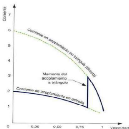
↑ Figura 4.36. En el instante del arranque, al conectar el motor en estrella, la corriente disminuye 3 veces la que consumiría si el arranque se hiciera de forma directa.
