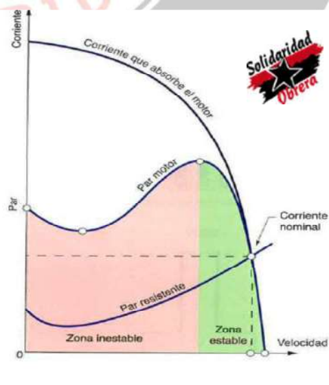
↑ Figura 4.32. Curva de corriente sobre la curva Par-Velocidad.
