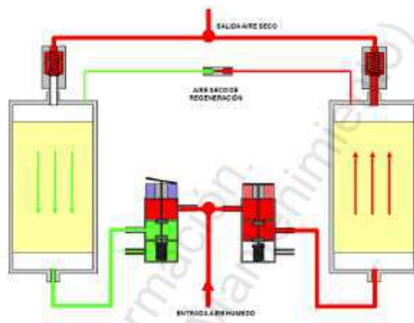
Figura 4-12. Secador.
