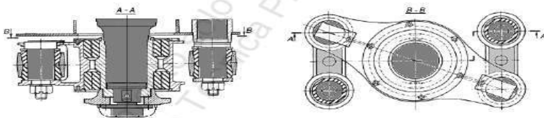
Figura. 2-52: Unión Watts
