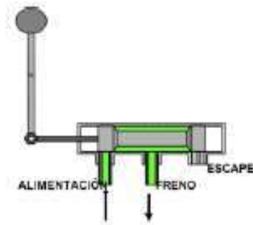
Figura. 5-1 Válvula de freno directo
