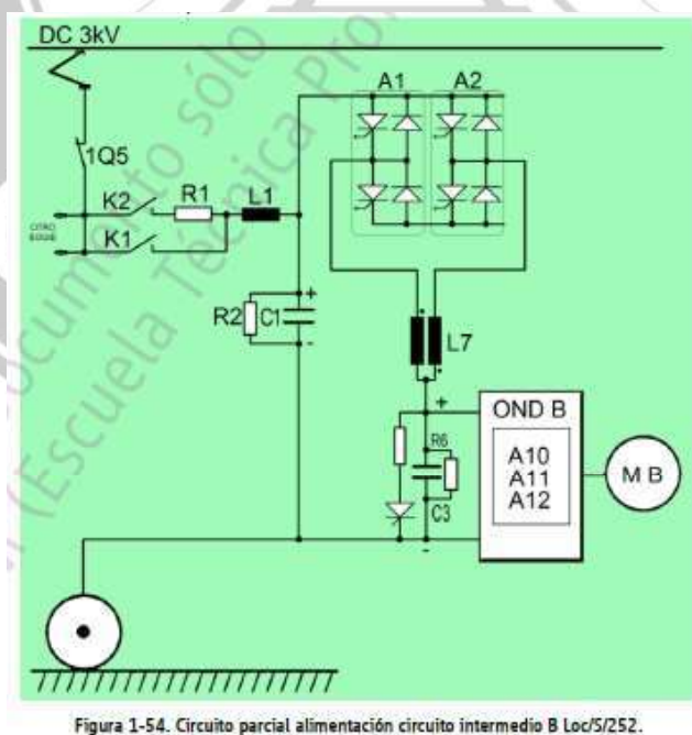
Figura 1-54. Circuito parcial alimentación circuito intermedio B Loc 5/252.
