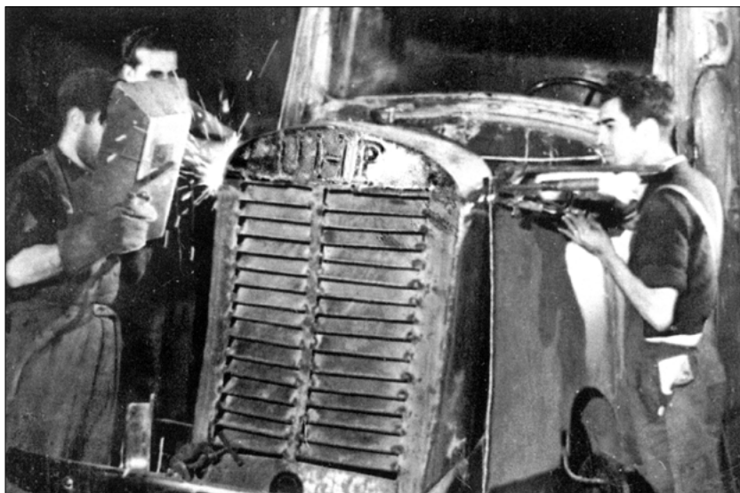
Blindaje con las siglas UHP en la Hispano-Suiza
